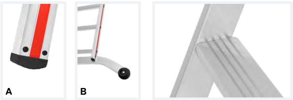
A Tacos interiores atornillados B Traviesa curvada
